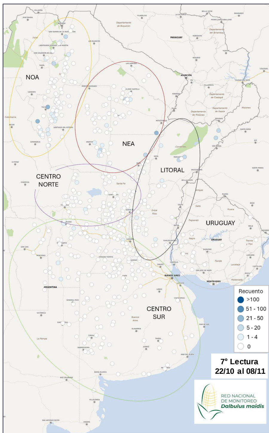
Figura 4. Captura de adultos de D. maidis /trampa, en función de la escala establecida con tonalidad en la gama de azules para la 7° lectura (22/10 al 08/11).
