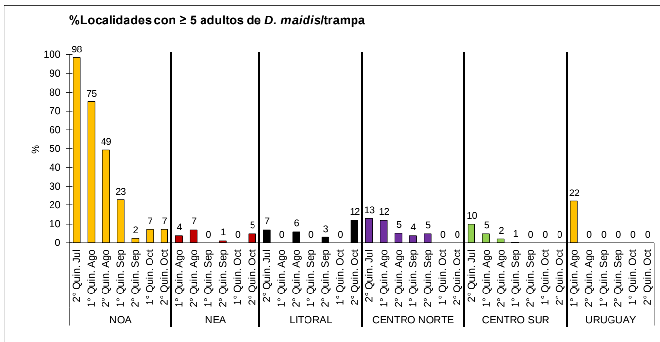
Figura 3. Evolución del porcentaje de localidades para cada región con cantidades \geq 5 adultos de Dalbulus maidis /trampas. Se detalla los porcentajes para cada quincena correspondiente a los informes de la Red Nacional de Monitoreo de la chicharrita del maíz ( Dalbulus maidis ).
